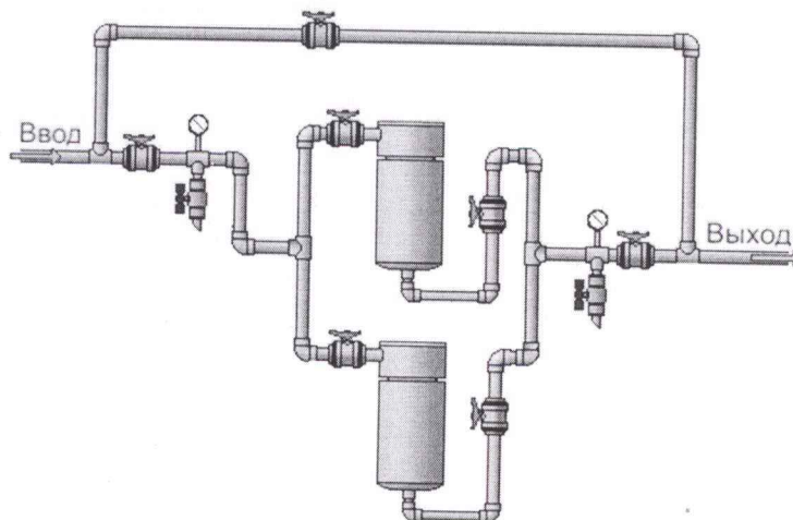
Принципиальная схема
